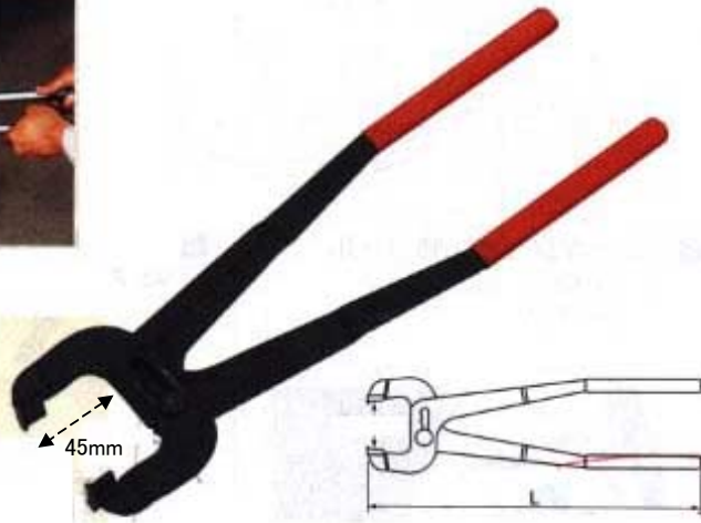
先端爪 24X14mm
