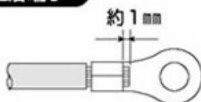
裸圧着端子
