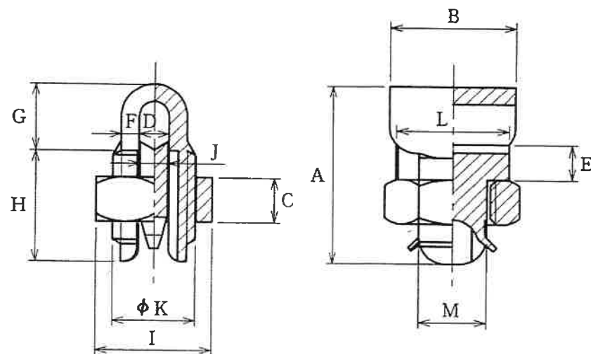
6B-11 ボルト型コネクタ
