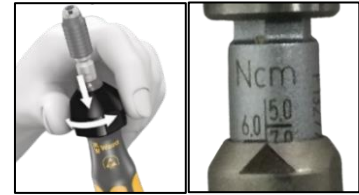
例) 6.0cNmに設定した状態 (画像はEA550MT-7)
