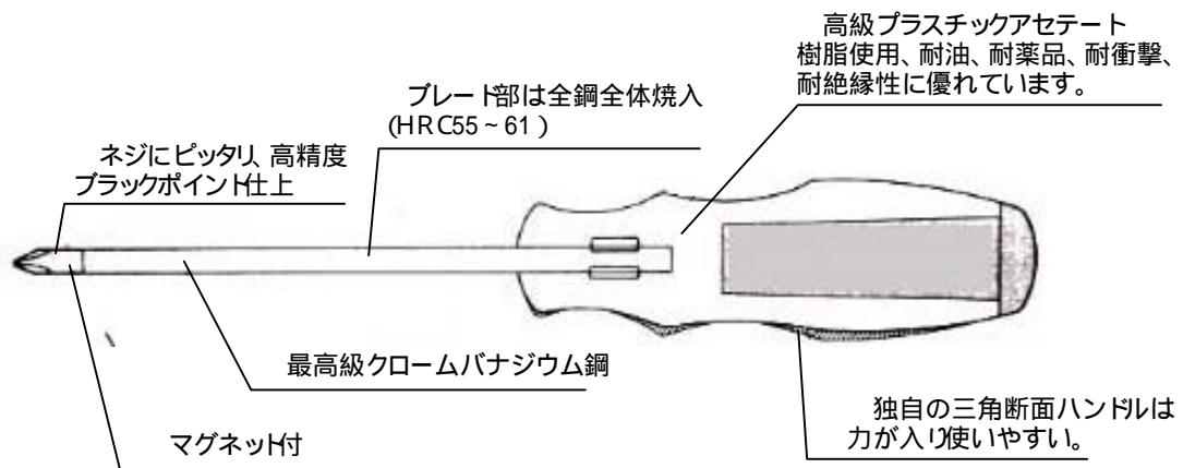
トルクを確実に伝え力がある三角形状
