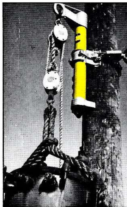
(使用例)
