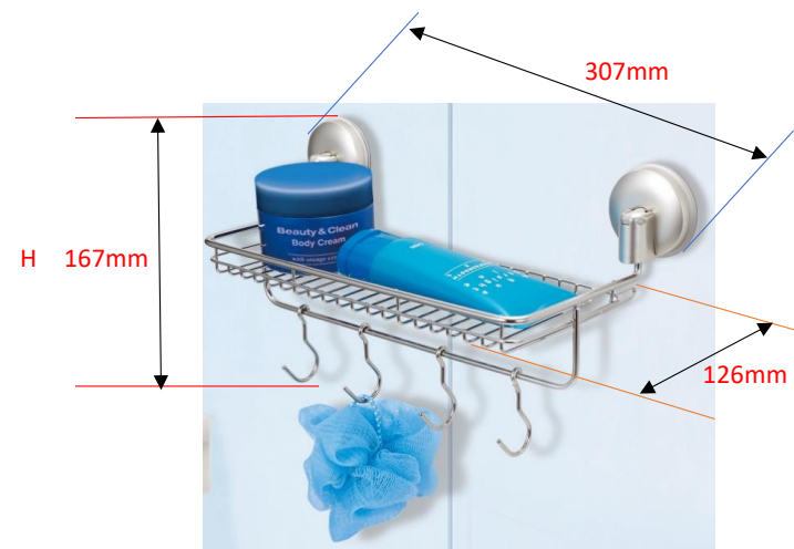
EA638LA-122 W307 × D126 × H167
