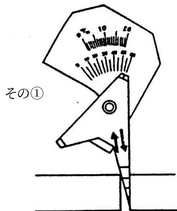
スキ間 小穴径 (3.5mm以下) の測定
