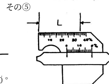
長さの測定 (40mm以下)
