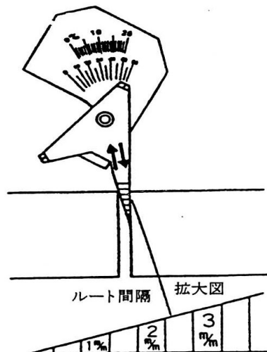
ルート間隔 (隙間) の測定
