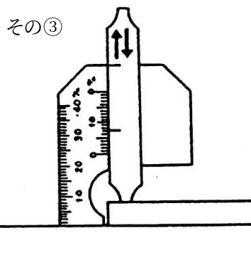
段差 板厚 (20mm以下) の測定
