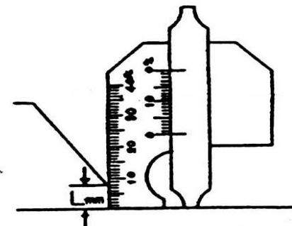
ルートフェースの測定
