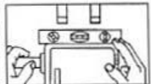
ヒューズボックスの据付
