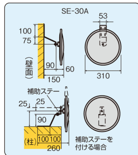
〈取付け図〉〈構造図〉
