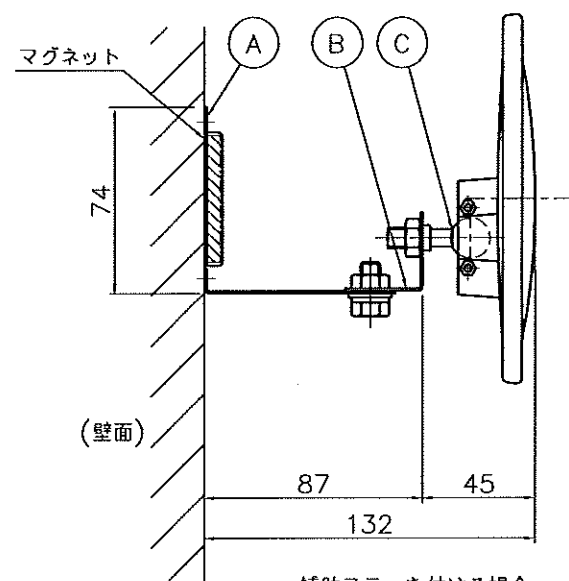
補助ステーを付ける場合
