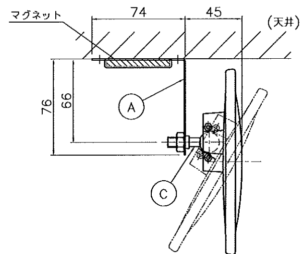
天井取付図
