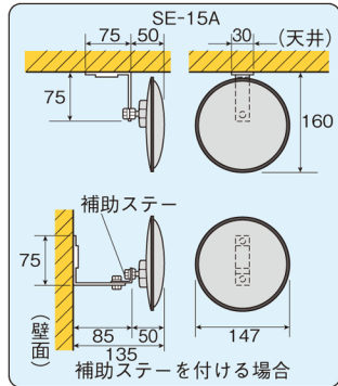
〈取付け図〉〈構造図〉
