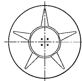
2 バックプレート (S=1/10)
