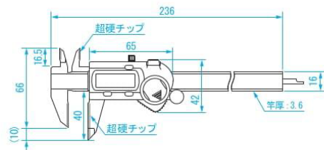
●寸法図
