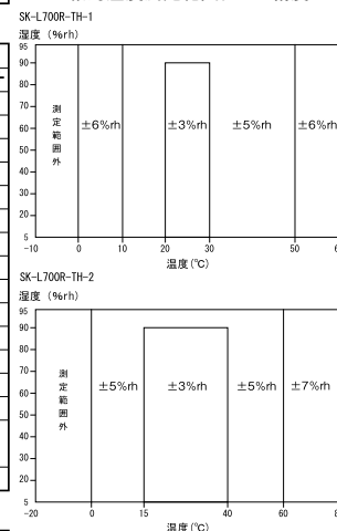
相対湿度測定範囲および精度
