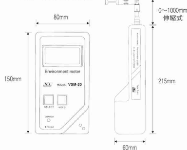
VSM-20 外観寸法図
