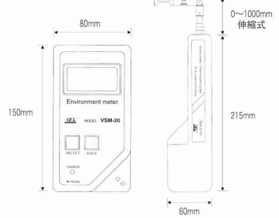
VSM-20 外観寸法図
