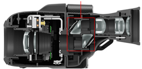
ポロプリズムI型
