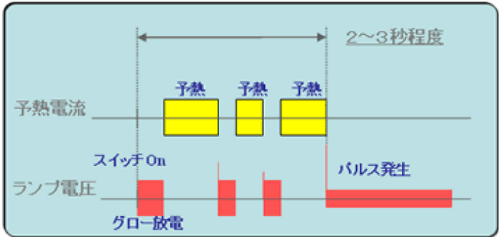
従来型点灯管
