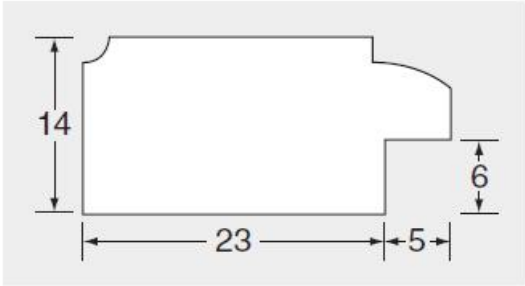
断面図
