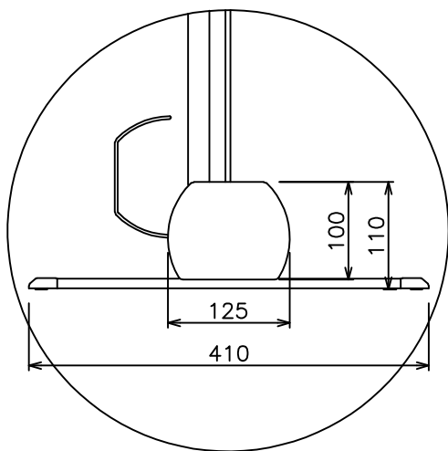
a部拡大図(S=1/5)
