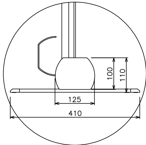
a部拡大図 (S=1/5)
