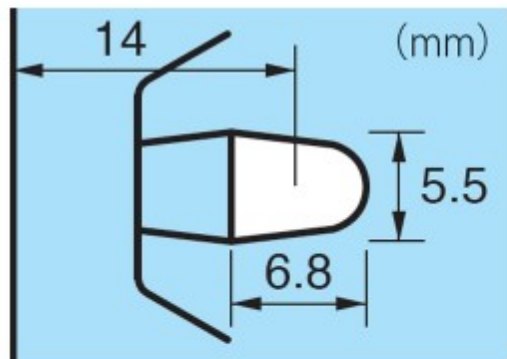
SL-112A とじ穴寸法
