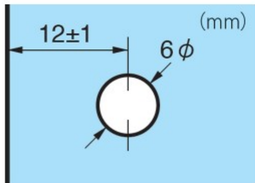
一般的な穴あけパンチ（比較）
