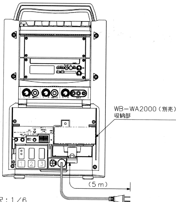
正面図
