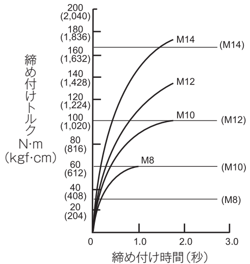
高力ボルト
