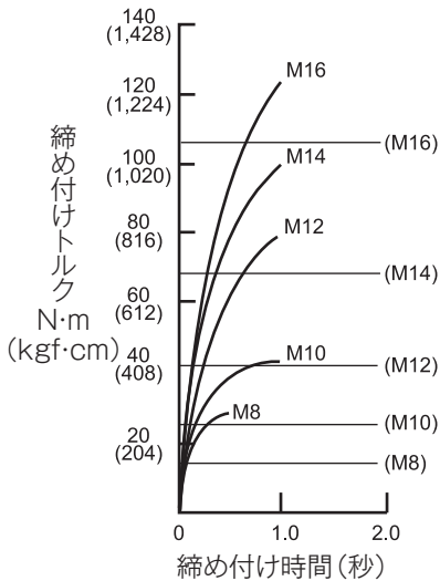
普通ボルト
