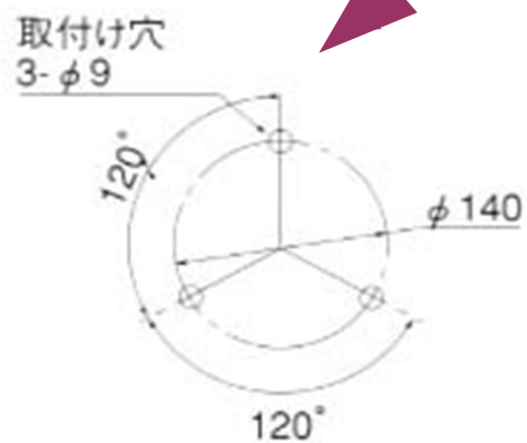
取付寸法図 (mm)
