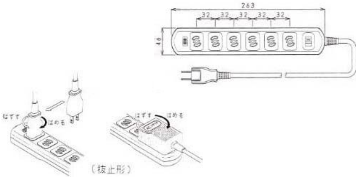
■寸法図
