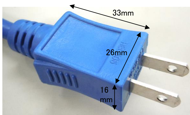
ストレートコンセント(-10、-20)
