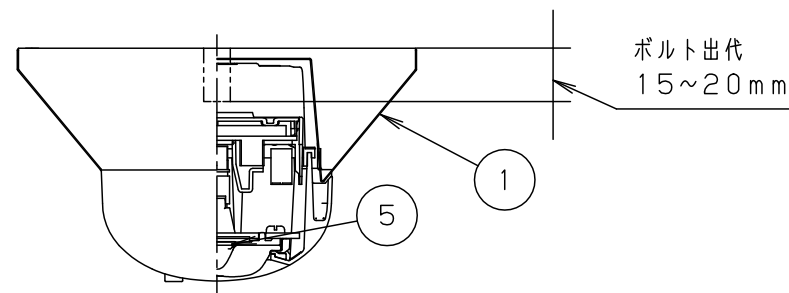
断面詳細図
