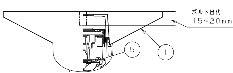
断面詳細図
