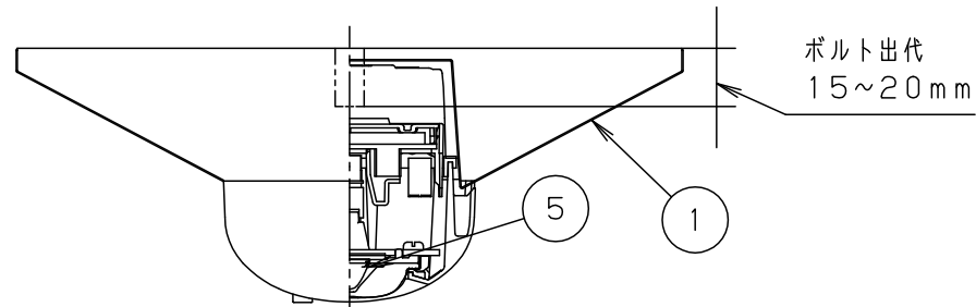
断面詳細図
