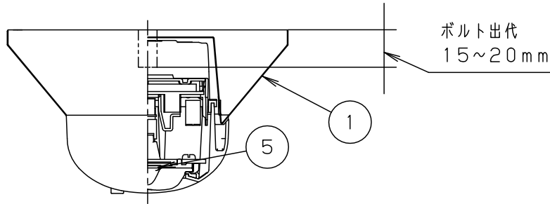
断面詳細図
