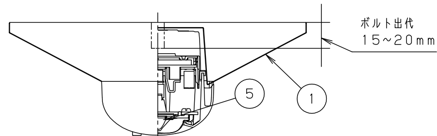
断面詳細図
