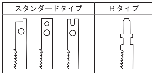
取付可能なブレードタイプ
