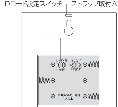
電池BOX
