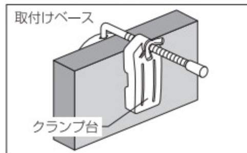
上からの取り付け
