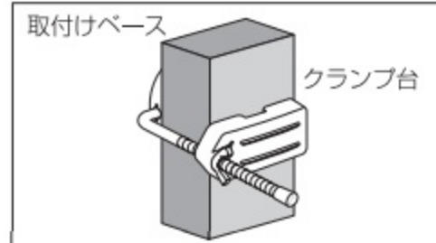
横からの取り付け
