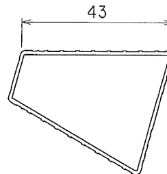
踏絛断面図 (1/1)
