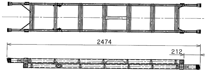
縮長時
