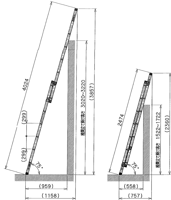
設置図 (1/30)
