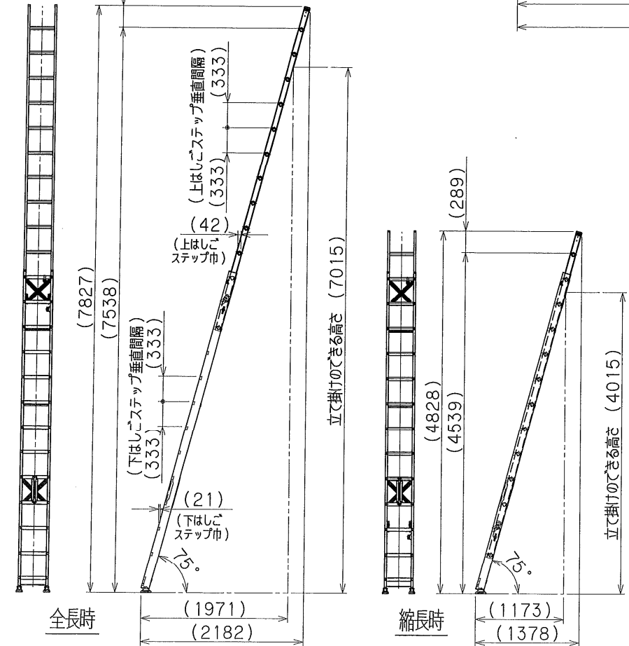
立て掛け寸法図 (1/50)
