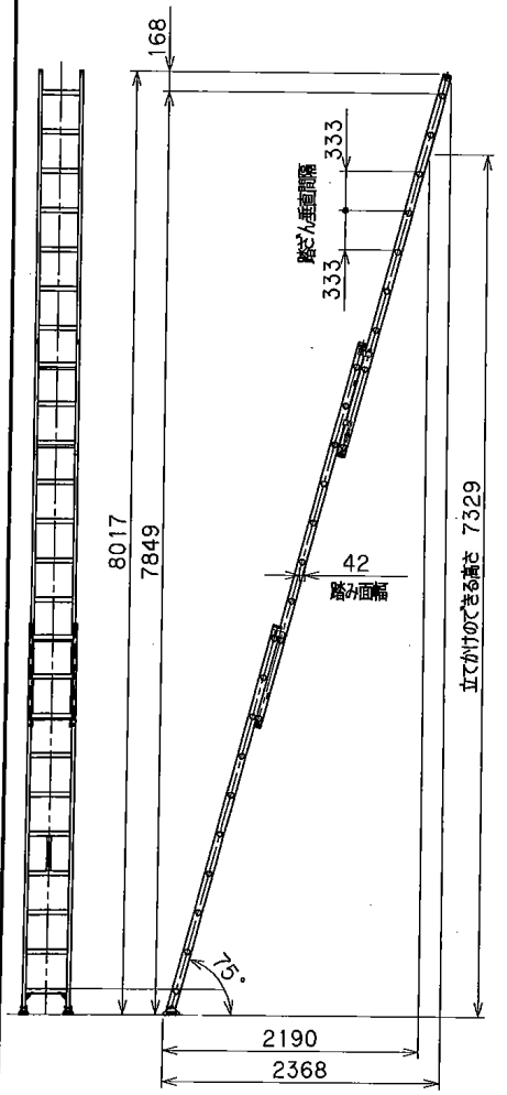
立てかけ寸法 (1/50)
