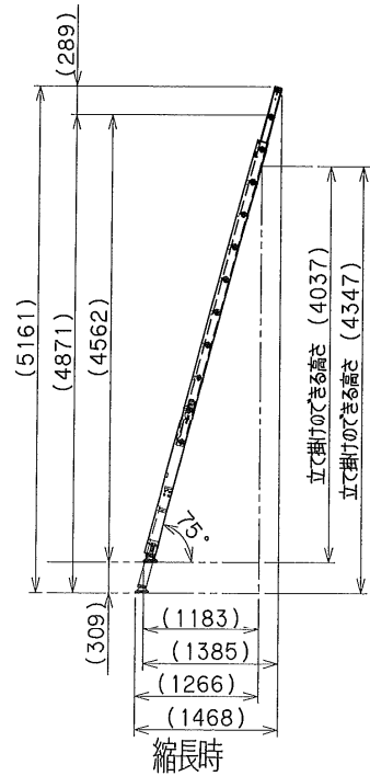
立て掛け寸法 (1/60)
