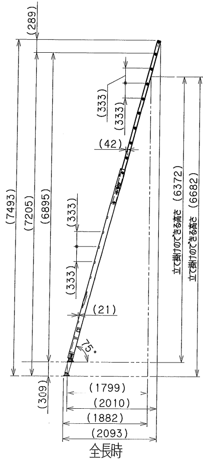
立て掛け寸法 (1/60)
