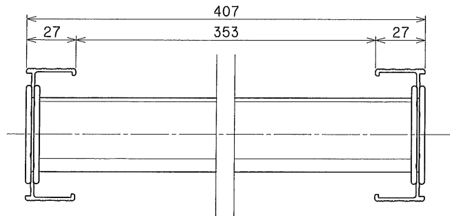
A-A断面
