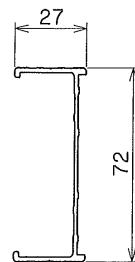
支柱
