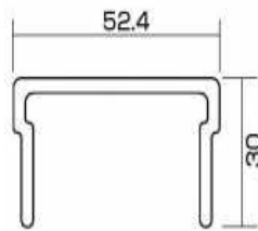
支柱形状
