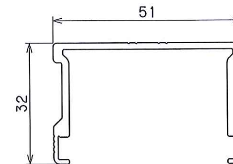
支柱断面図 (1/1)
