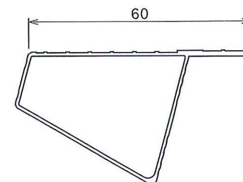
踏ざん断面図 (1/1)
