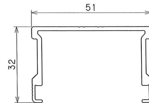
支柱断面図 (1/1)
