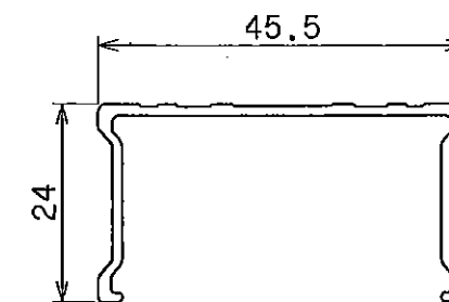
支柱(1/1)
