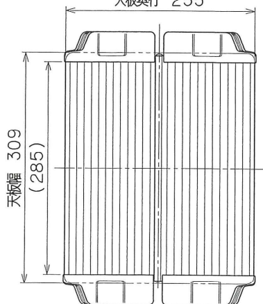
A 矢視図
