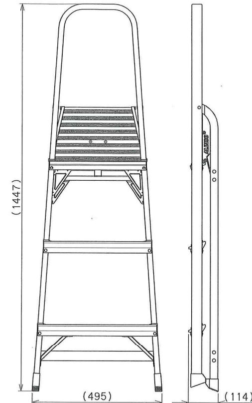
収納状態
