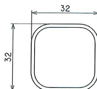
手すり材 (1/1)
