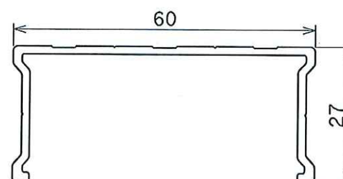
背面支柱 (1/1)
