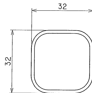
手すり材
