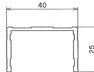
支柱
